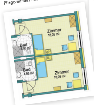
Der Grundriss zeigt das Beispiel eines 1-Bett-Pflegezimmers mit einer Größe von 21 m 2 .
