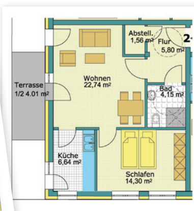
Der Grundriss zeigt eine Wohnung im Betreuten Wohnen.
